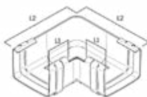
STŪRIS, (UNIVERSĀLS)
